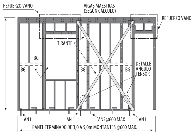
Elevación típica Muro MP2
