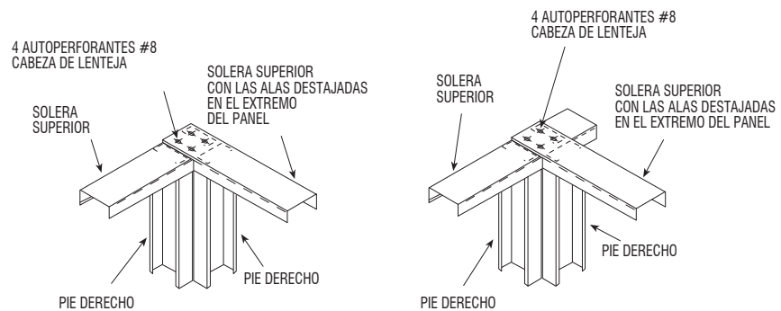
DETALLE TÍPICO DE ENCUESTRO DE SOLERAS SUPERIORES
