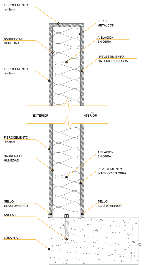
CORTE VISTA CAPAS ANTEPECHO PREF.
