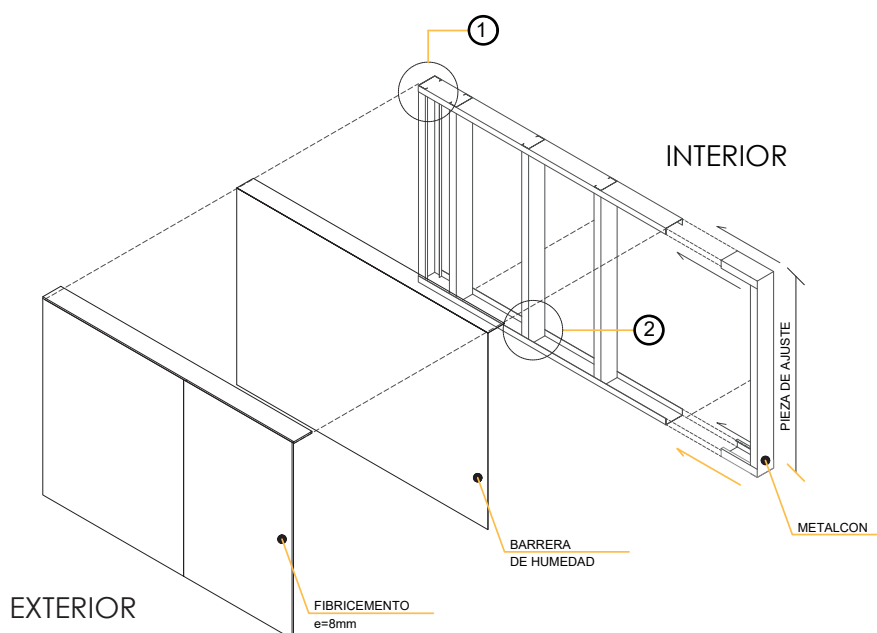
ISOMETRICA CAPAS ANTEPECHO PREFABRICADO
