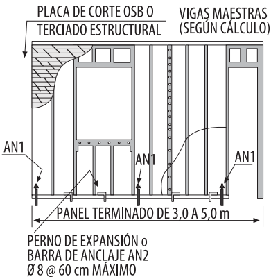
Elevación típica Muro MP1
