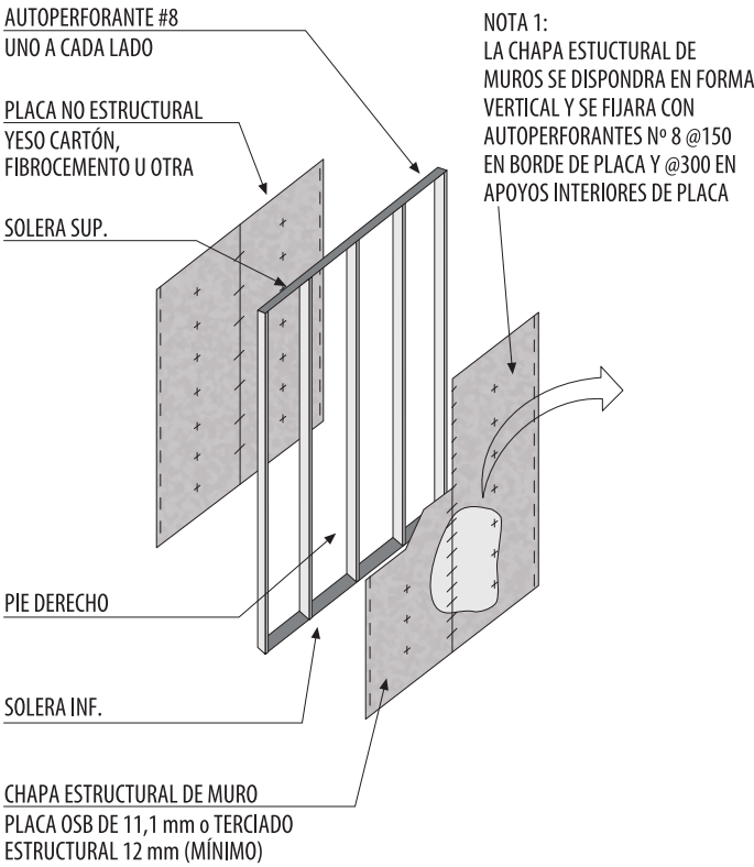
Elevación típica Muro MP1
