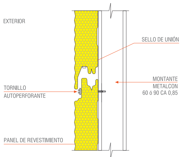
Revestimiento Aislado / Friso
