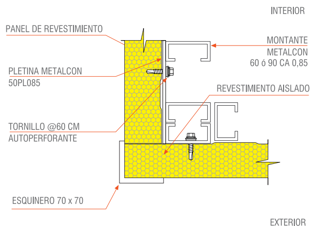
Revestimiento Aislado / Canto Recto
